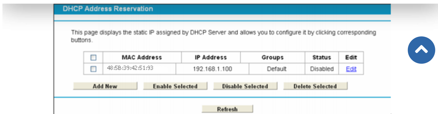
Рис. 5. Созданное правило для статического IP адреса
